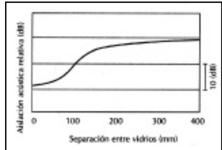
Fig. 5.5: influencia del ancho de cámara en la aislación acústica de un DVH (fuente: BI n°19 VASA)
