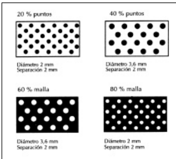
Fig 3.3: diseño standards de vidrios serigrafiados (Fuente: BI n° 11 VASA)
