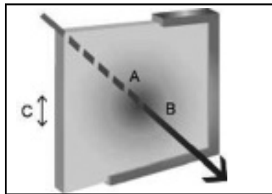
Fig. 7.1: Generación de tensión térmica A: Caliente, trata de expandirse B: frío, resiste la expansión C: tensión de tracción (fuente: BI n° VASA)
