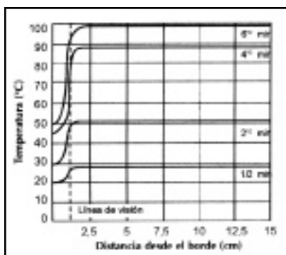
Fig.7.4: influencia de la altura del marco en el stress térmico (fuente: BI nº 21 VASA)
