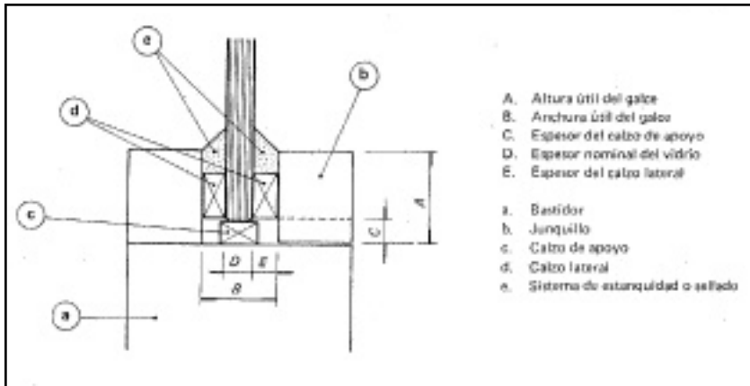
Fig. 8.2: elementos que intervienen en una correcta instalación
