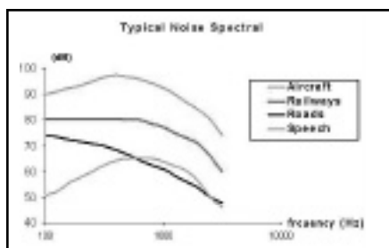
Fig. 5.2: espectro de frecuencia típicos (aproximados) para distintas fuentes de ruidos
