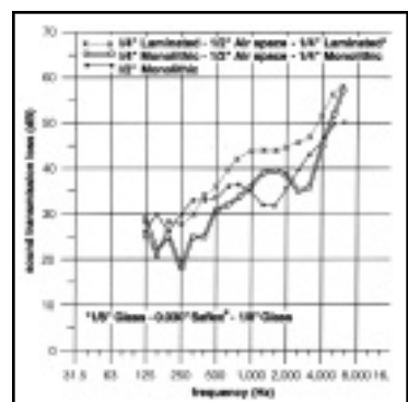
Fig. 5.6: absorción acústica de un vidrio monolítico de 12mm, un DVH 6/12/6 y un DVH 3+3/12/3+3. (fuente: Acoustical Glazing Design Guide - Saflex)
