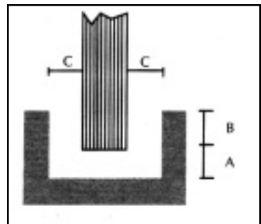
Fig. 8.13: luces de acristalamiento (BI VASAnº13)
