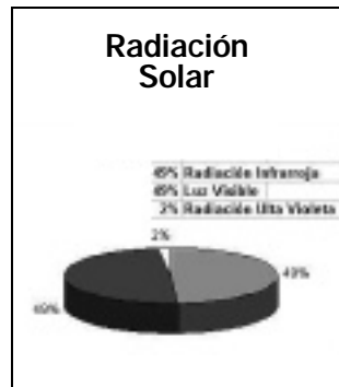
Fig. 4.6: composición de la radiación solar
