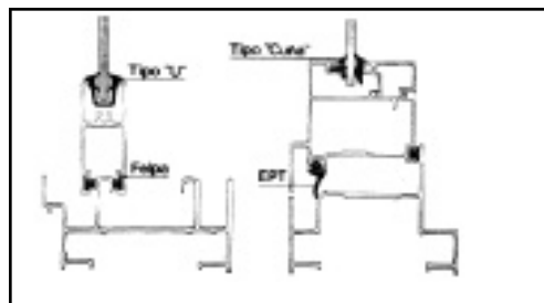
Fig. 9.1: burletes tipo "U" y tipo cuña
