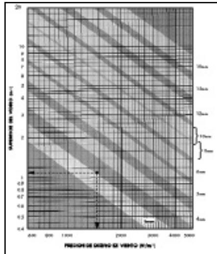
Fig. 10.2: Doble Vidriado Hermético, soportado en sus cuatro bordes
