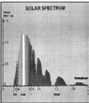
Fig. 4.5: Espectro de Radiación Solar
