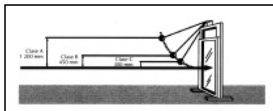
Fig 6.3: dispositivo de ensayo IRAM 12559 (fuente: BI n°14 VASA)
