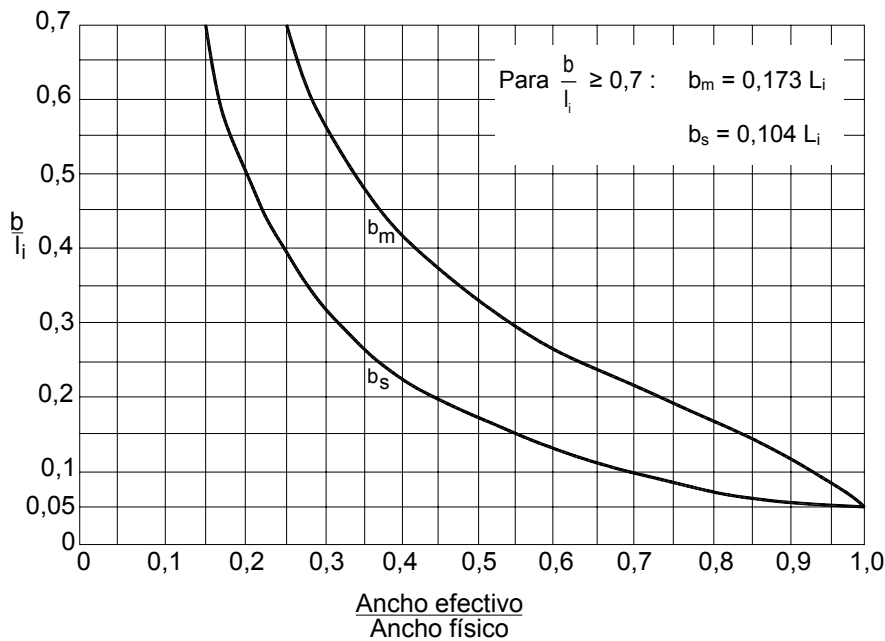
Figura 4.6.2.6.2-2 – Valores de los coeficientes de ancho de ala efectivo para b_m y b_s para los valores de b/l_i indicados
