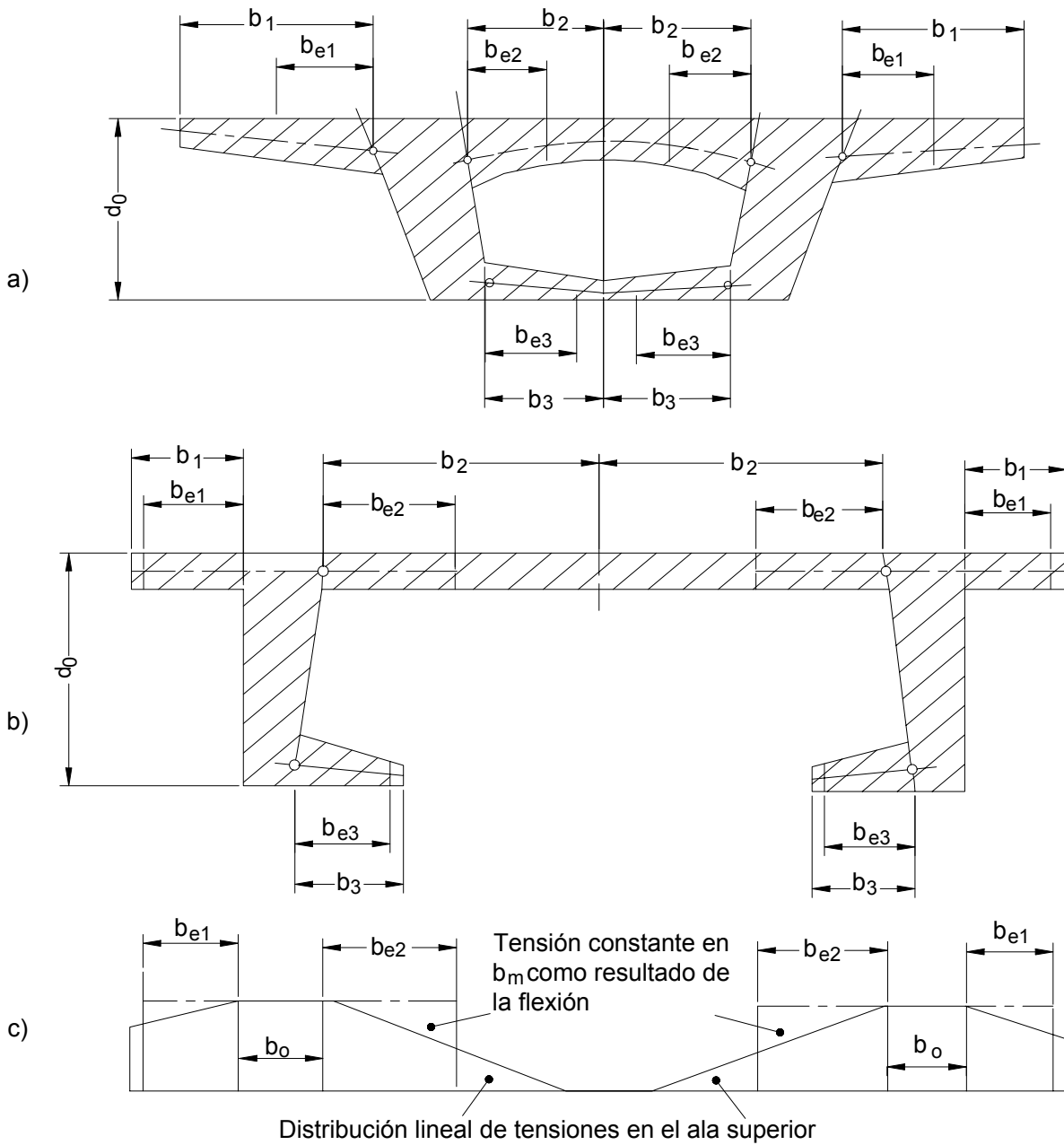
Figura 4.6.2.6.2-3 – Secciones transversales y anchos de ala efectivos correspondientes, b_e , para flexión y corte
