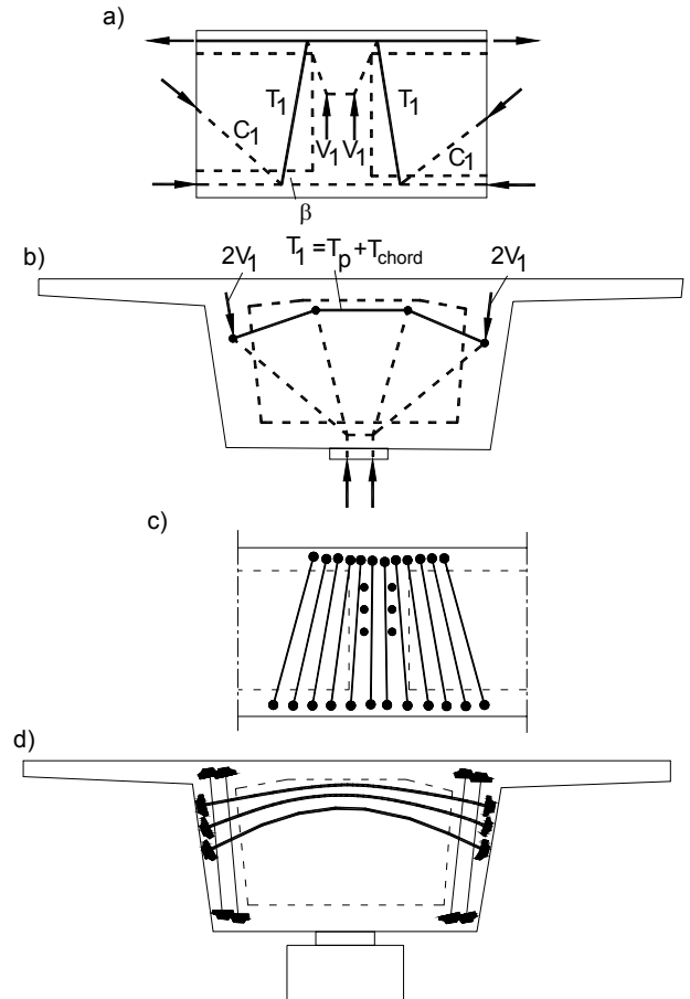
Figura C5.13.2.2-1 – Diafragma de un puente tipo viga cajón: a) Regiones perturbadas y modelo del alma cerca del diafragma; b) Diafragma y modelo; c) y d) Pretensado del alma y el diafragma (Schlaich et al., 1987)
