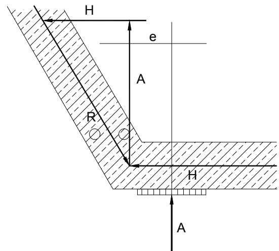
Figura C5.14.2.4.6c-2 – Reacción excéntrica en las placas de lanzamiento
