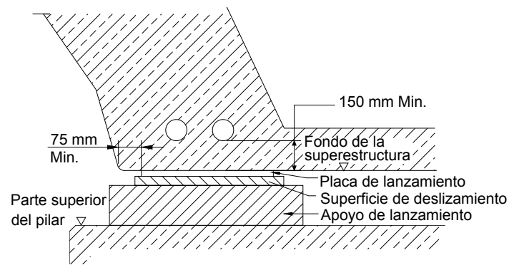
Figura C5.14.2.4.6c-1 – Ubicación de las placas de lanzamiento
