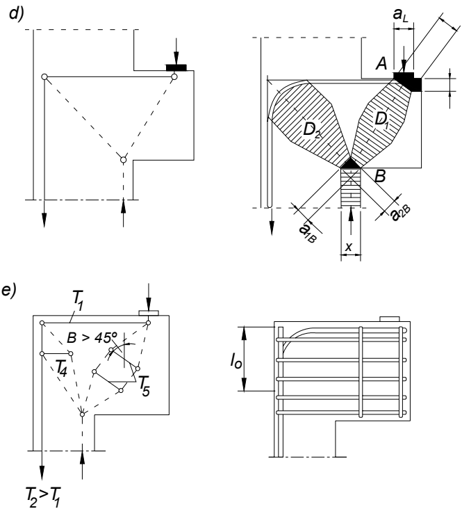
Figura C5.13.2.4.1-1 – Diferentes condiciones de apoyo que conducen a diferentes modelos de bielas y tirantes y diferentes disposiciones de armadura en las cartelas y resaltes horizontales tipo viga (Schlaich, 1987)
