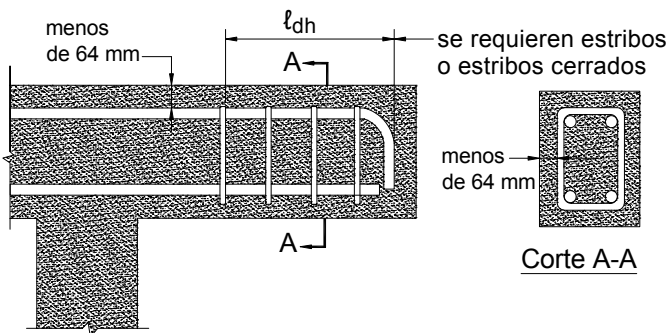
Figura 5.11.2.4.3-1 – Estribos para las barras terminadas en gancho
