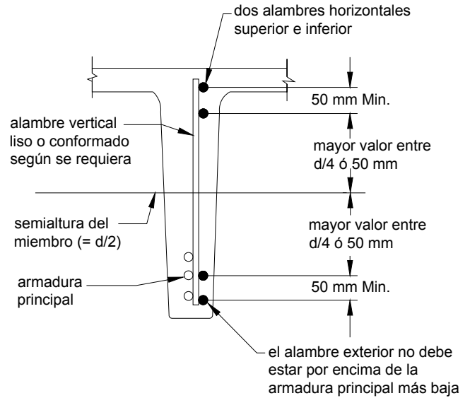
Figura C5.11.2.6.3-1 – Anclaje de armadura de corte en forma de malla de alambre soldado de una rama, ADI (1989)
