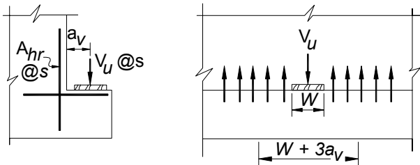
Figura 5.13.2.5.5 -1 – Armadura de suspensión en un resalto único
