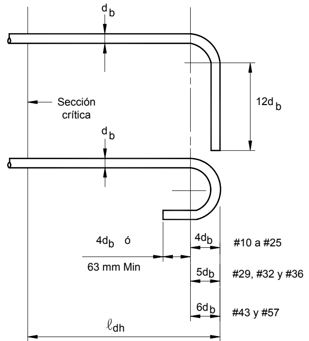
Figura C5.11.2.4-1 – Detalles de las barras terminadas en gancho para el desarrollo de ganchos normales (ACI)
