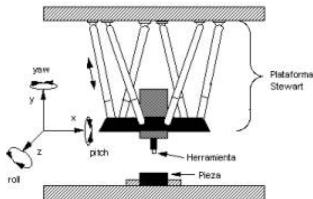
Fig. 2: Configuración básica de una máquina de arquitectura paralela (Plataforma Stewart).
