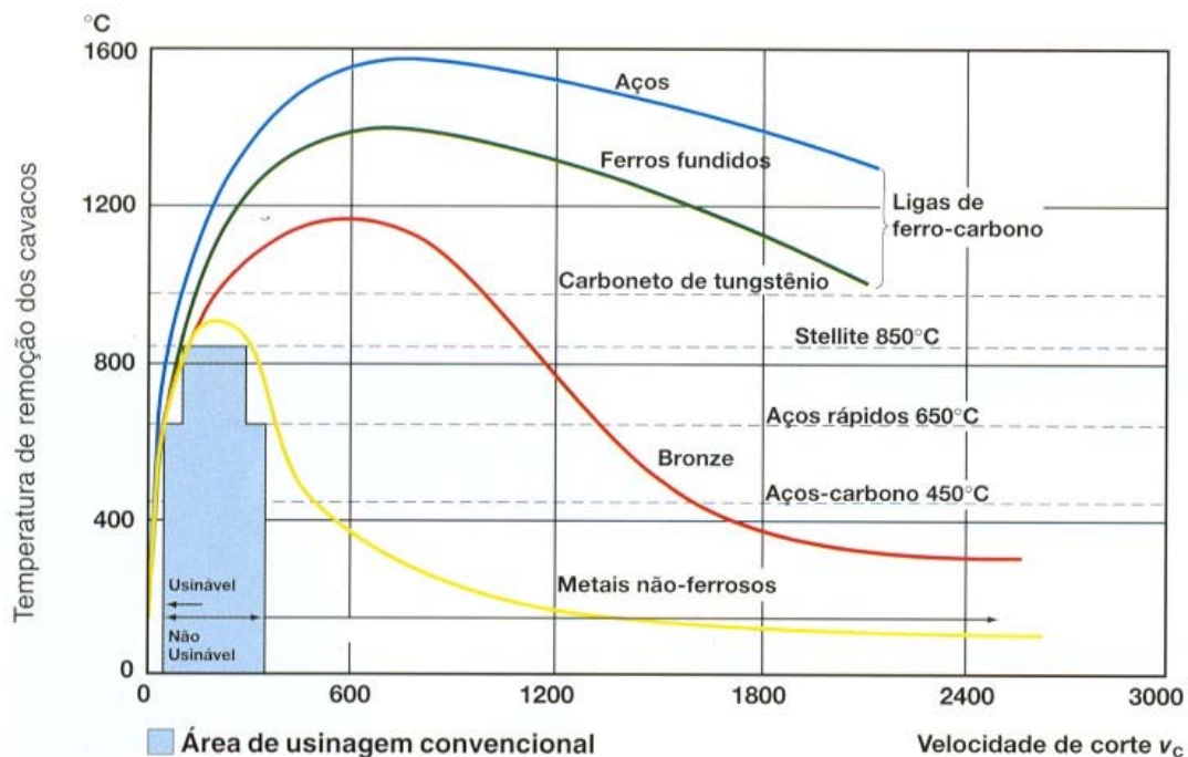
Fig. 1: Temperatura de formación de viruta (°C) vs. Velocidad de corte (m/min) .
