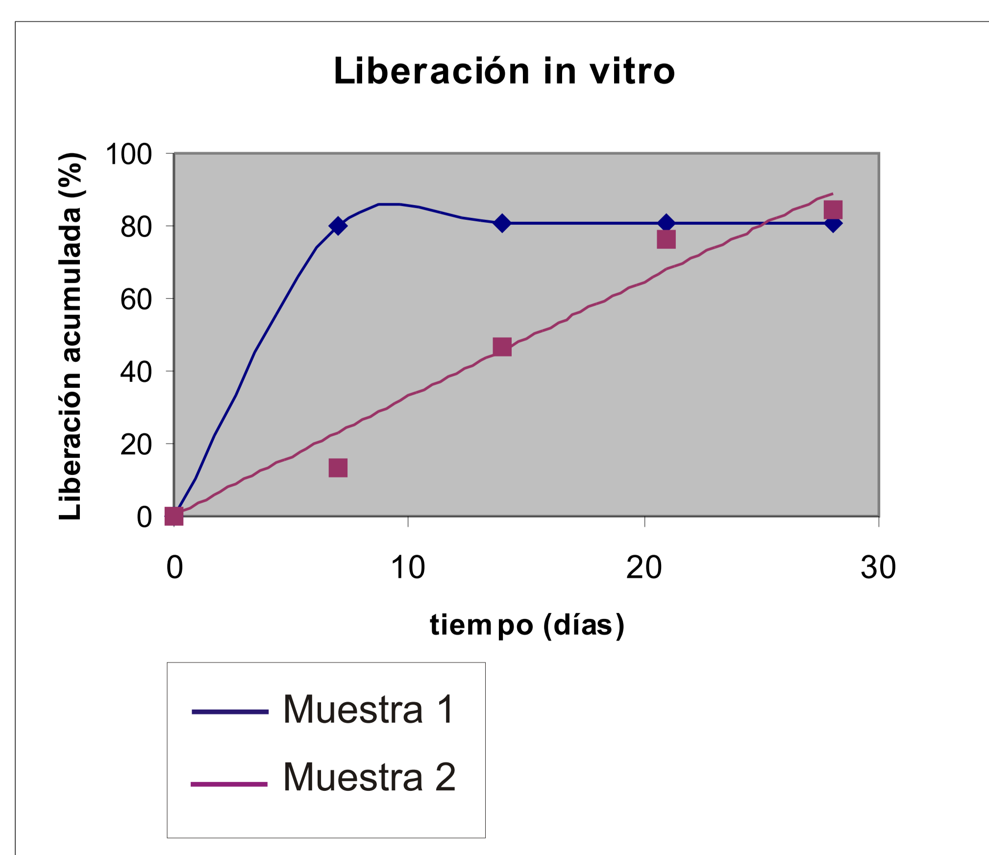
Figura 2 Curvas de liberación in vitro
